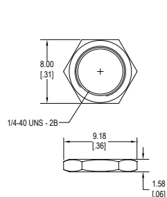
Hex Nut 1/4 - 40
